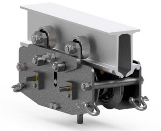
ATTREZZO PER INSERIMENTO FILO DI CONTATTO CONTACT WIRE INSERTION TOOL
