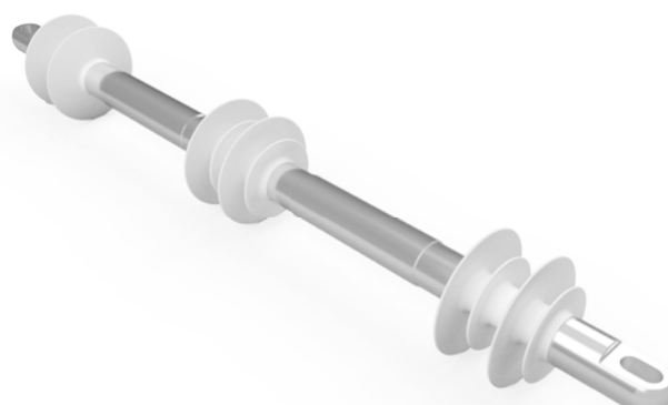
SOSPENSIONE PER SOVRAPPOSIZIONE ISOLATA INSULATED OVERLAP SUPPORT
